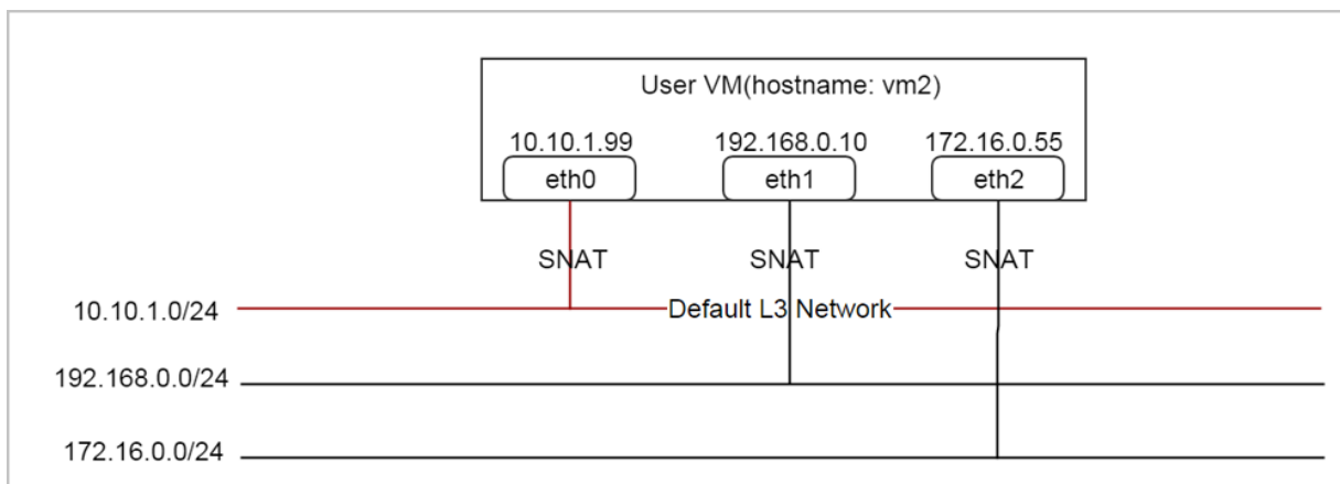
图 3: 用户云主机
