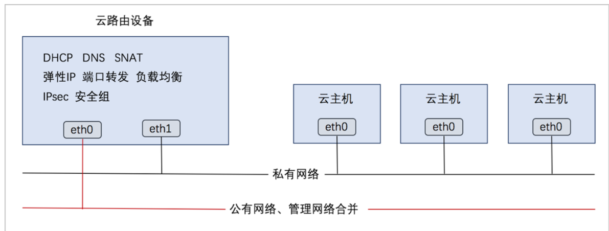
图 26: 部署方式-1
